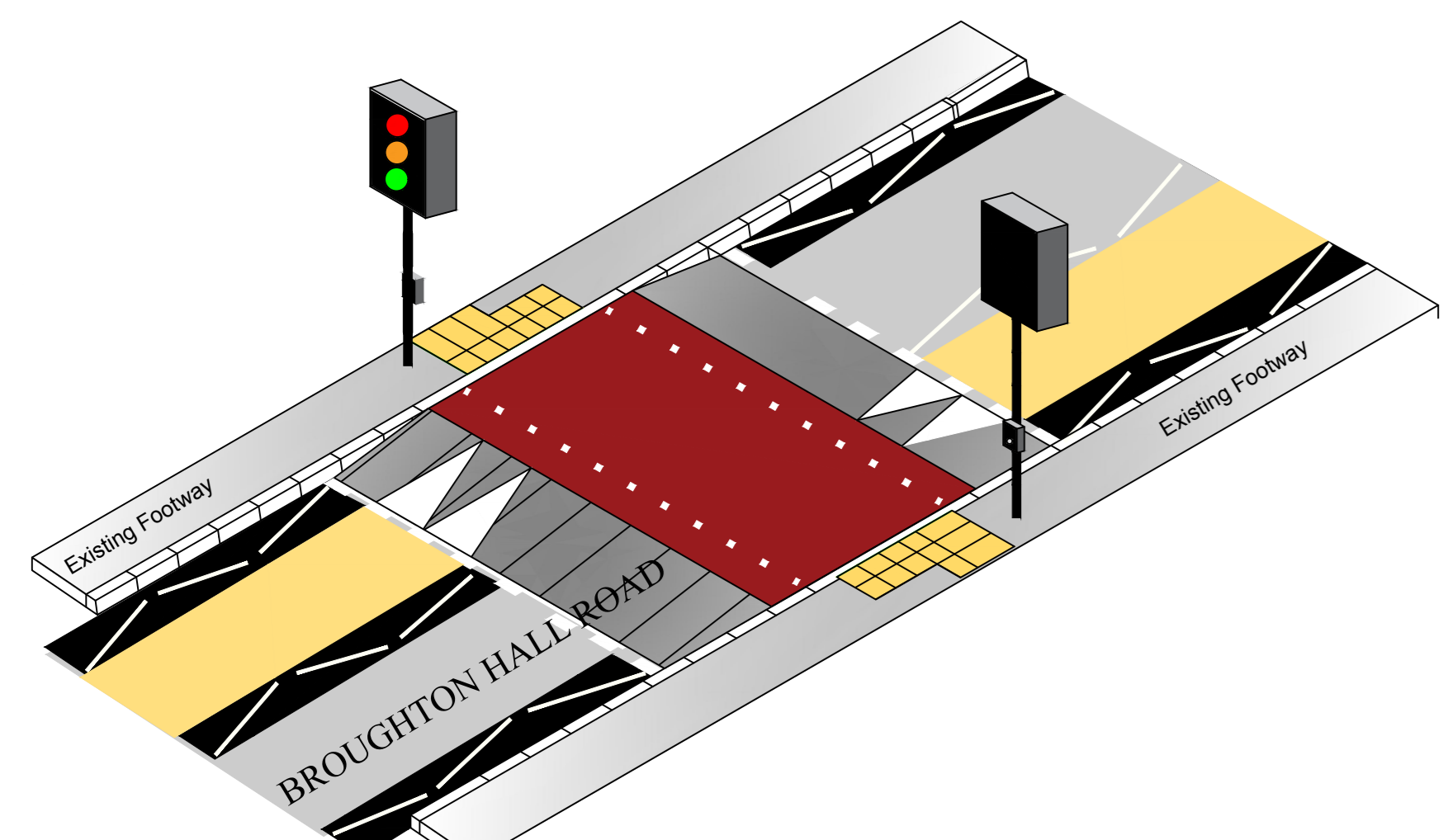
Croesfan pelican presennol wedi'i fowntio ar wyneb newydd wedi'i godi. Existing pelican crossing mounted on new raised table.
